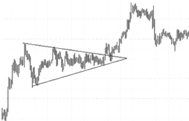
Рис. 1.20. «Вымпел»
