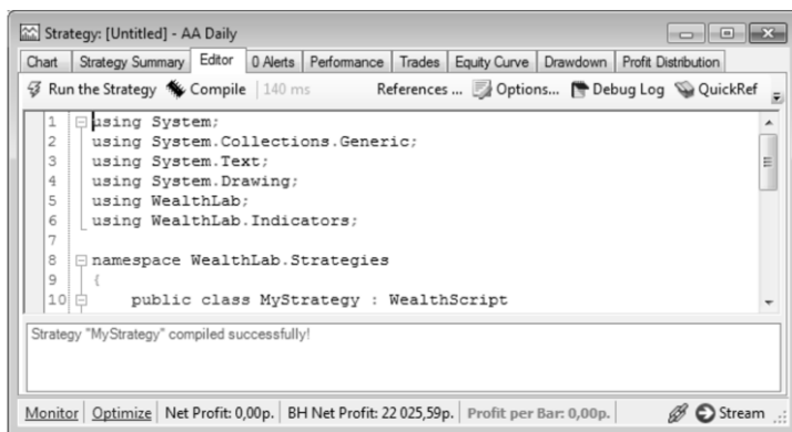
Рис. 5.14. Редактор стратегий
