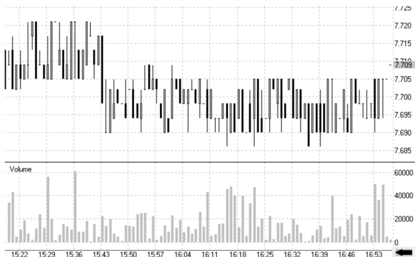
Рис. 1.21. Индикатор объема
