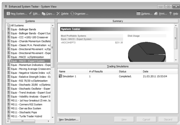
Рис. 5.4. Тестер систем
