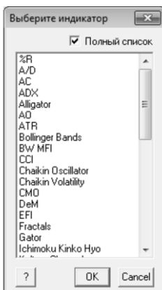
Рис. 2.12. Список индикаторов
