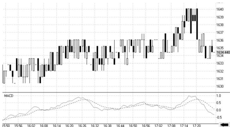
Рис. 1.27. Индикатор MACD
